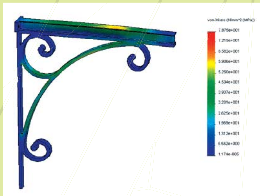
Calcul d'une pièce de ferronnerie
