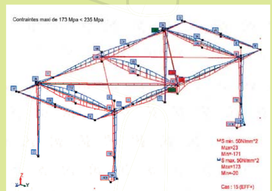
Calcul de structure charpente
