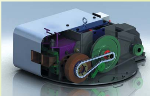
Broyeur de rives sur SOLIDWORKS
