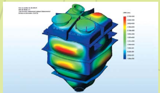
Calcul réservoir
