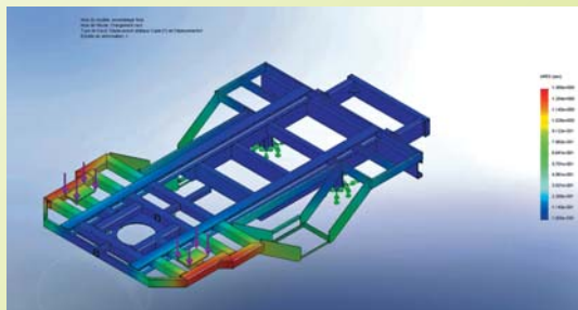
Calcul d'un châssis de remorque
