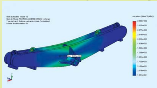
Calcul d'un palonnier
